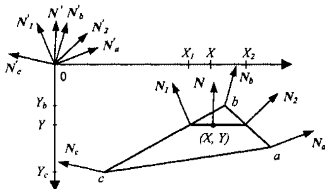
Рис. 4.39. Интерполяция векторов нормалей
