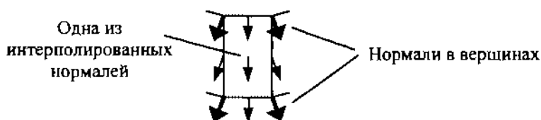
Рис. 4.41. Интерполяция нормалей дает более точный результат
