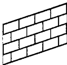
Аксонометрическая проекция
