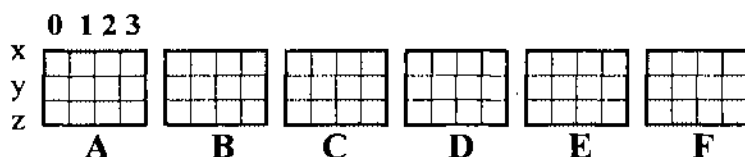
Рис. 4.4. Отдельные грани
