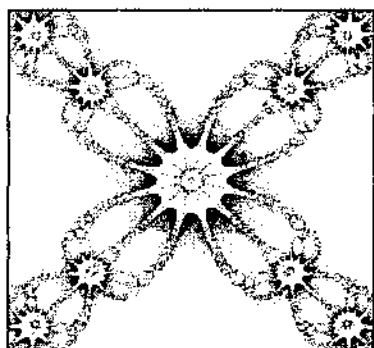
Рис. 3.31. Фрактал Ньютон
