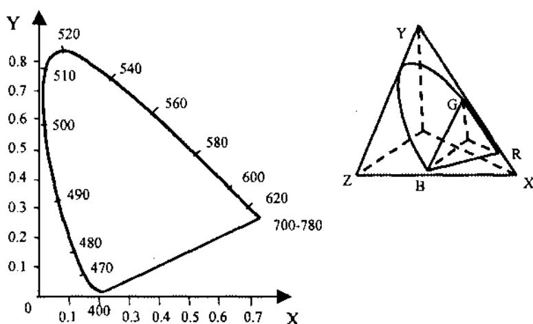
Рис. 1.30. Цветовой график для модели МКО XYZ
