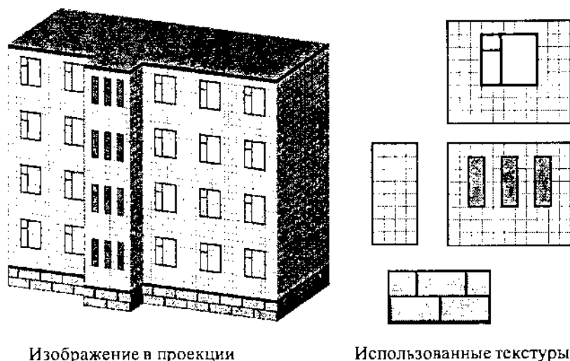
Рис. 3.29. Блочное текстурирование
