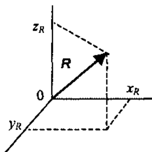
Рис. 4.31. Радиус-вектор
