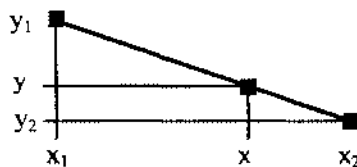
Рис. 3.1. Отрезок прямой
