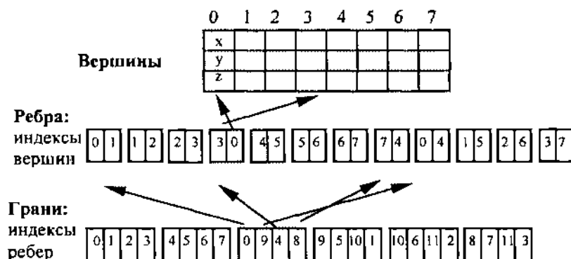
Рис. 4.7. Линейно-узловая модель
