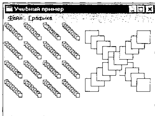
Рис. 6.2. Пример метафайла
