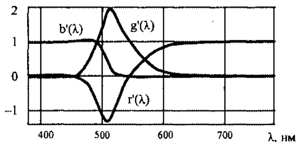
Рис. 1.25. Трехцветные коэффициенты смешивания RGB
