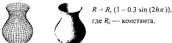
Рис. 5.42. Сетка граней и закрашивание методом Гуро
