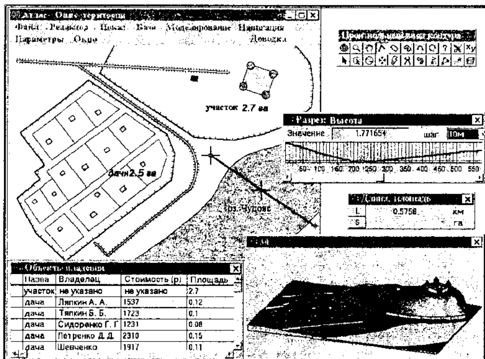
Рис. 2. Работа с геоинформационной системой (ГИС "ОКО")
