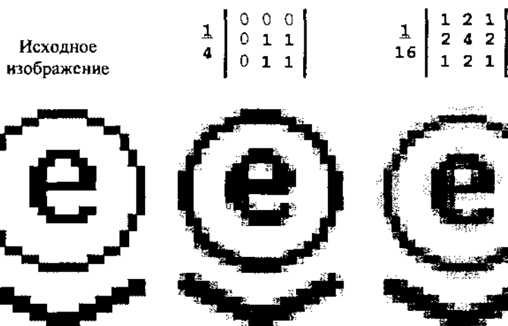
Рис. 1.35. Два сглаживающих фильтра с маской 3 \times 3
