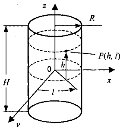
Рис. 5.28. Цилиндр
