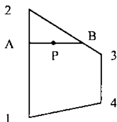
Рис. 3.28. Полигон
