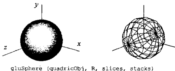
Рис. 10.5. Шар
