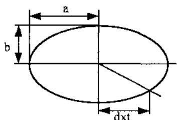
Рис. 3.5. Вывод эллипса
