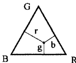
Рис. 1.22. Треугольник Максвелла
