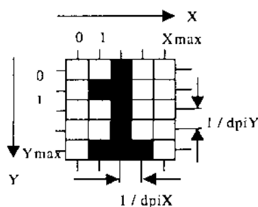
Рис. 1.1. Растр
