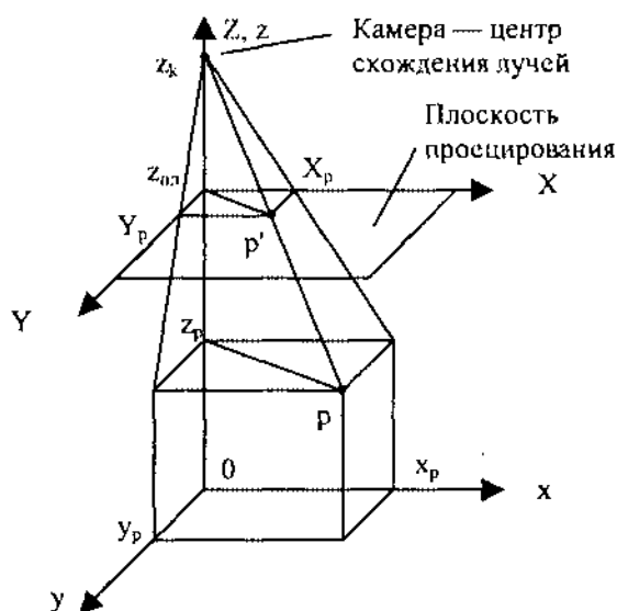
Рис. 2.17. Перспективная проекция
