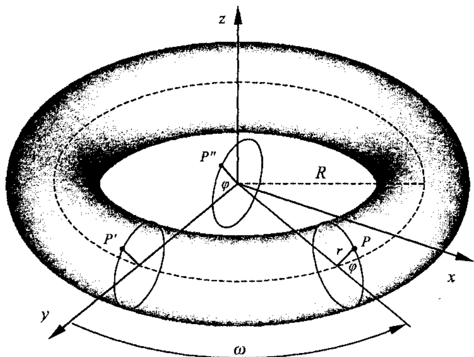
Рис. 2.14. Тор
