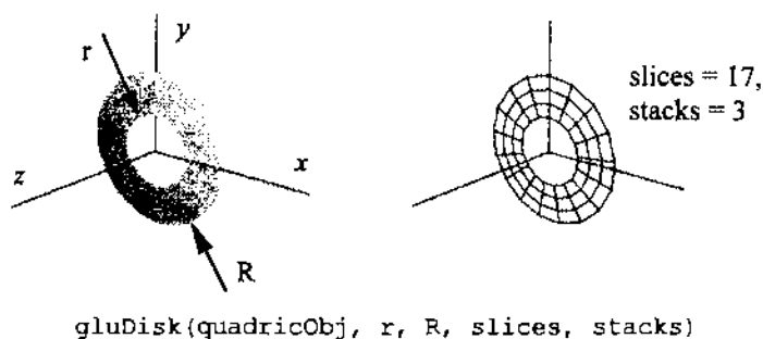
Рис. 10.6. Диск
