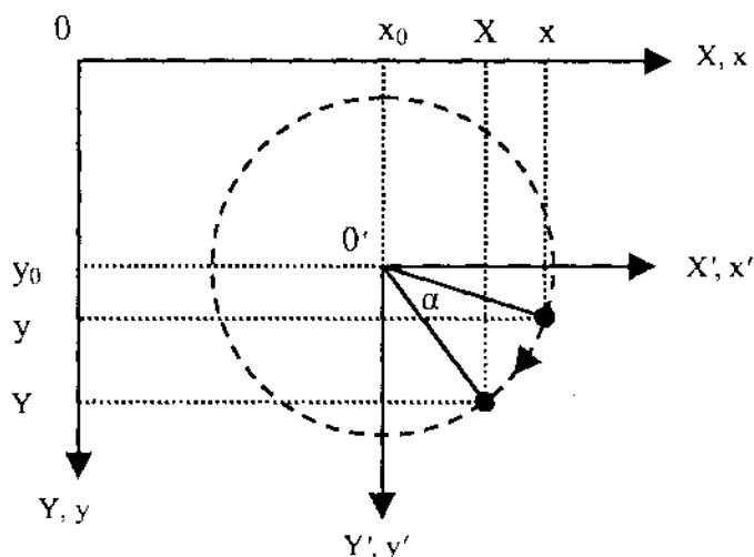
Рис. 2.13. Вращение вокруг произвольного центра
