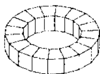
Рис. 5.49. Кольцо
