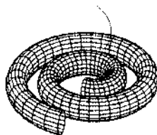
Рис. 5.50. Спираль
