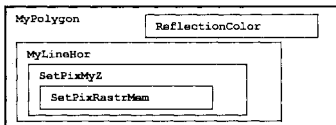
Рис. 8.6. Вложенность функций
