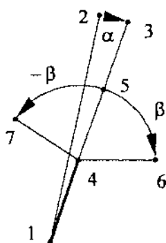
Рис. 3.33. Опорные точки элементов фрактала
