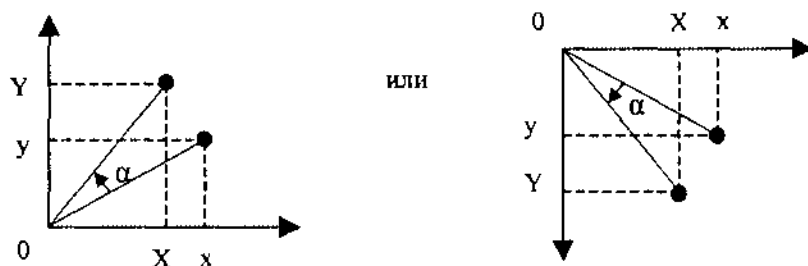
Рис. 2.9. Поворот объекта
