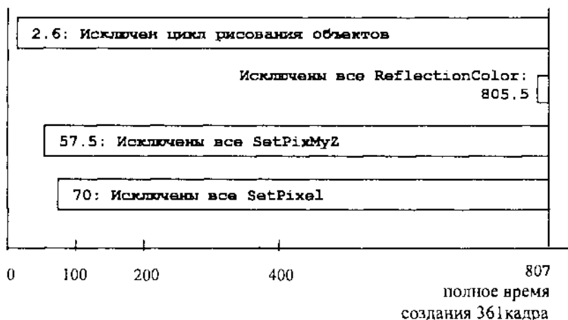
Рис. 8.3. Диаграмма исключения операций
