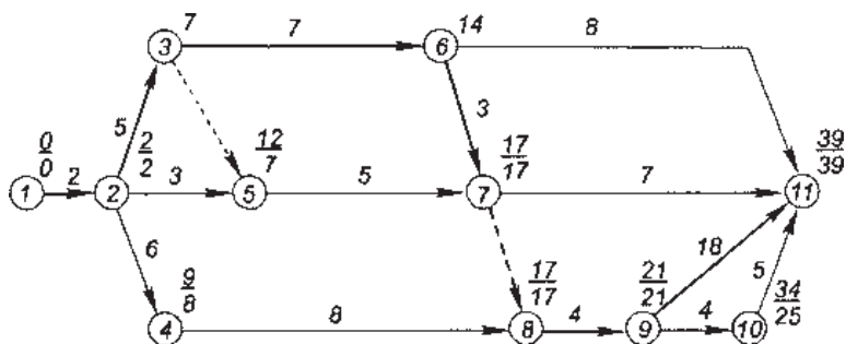
Рис. 11. Сетевой график
