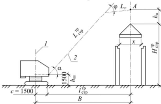
Рис. 3. Подбор стрелового крана
